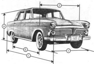
Fig. 1. AERO-WILLYS 2400 — modelo 3-1145
