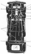
Chassi de Rural 4 x 2 (8122 e 8126)
