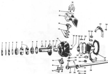
EIXO (MUNHÃO) DIANTEIRO
