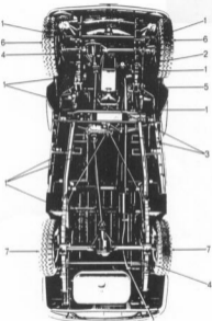
Chassi de Rural 4 x 4 (8222)
