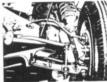
Suspensão independente — modelo 9122.
