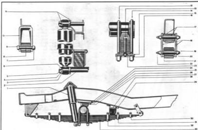
MOLAS DIANTEIRAS
