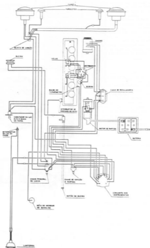
DIAGRAMA DO SISTEMA ELÉTRICO JEEP UNIVERSAL E JEEP 101
