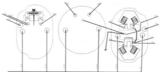
Fig. 9. Esquema das ligações dos instrumentos
