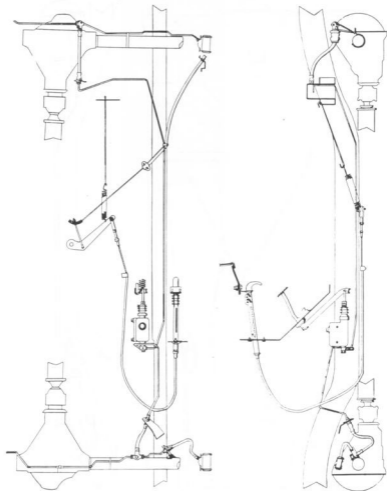
INSTALAÇÃO DO FREIO — JEEP UNIVERSAL E MODELO 101
