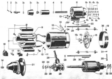
MOTOR DE PARTIDA "WALITA"
