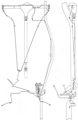
INSTALAÇÃO DO FREIO — AERO-WILLYS
