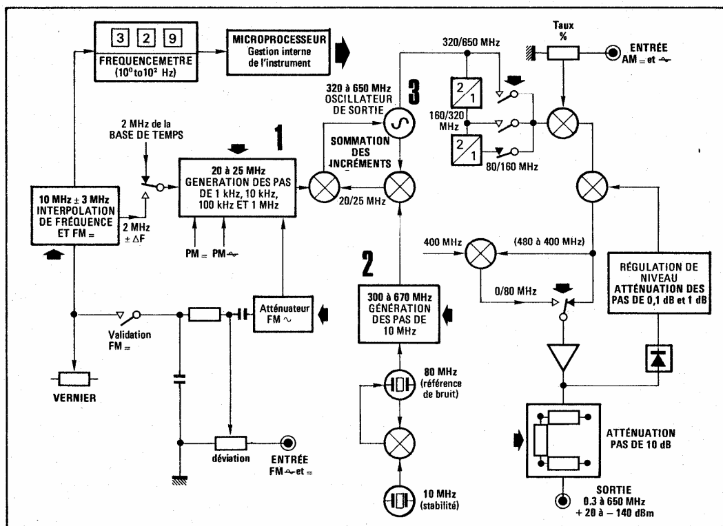
Figure 4-1 : PRINCIPE DE FONCTIONNEMENT DU 7100
