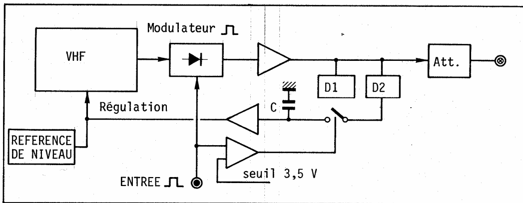
Figure 4-6 : PRINCIPLE DE LA MODULATION PAR IMPULSIONS
