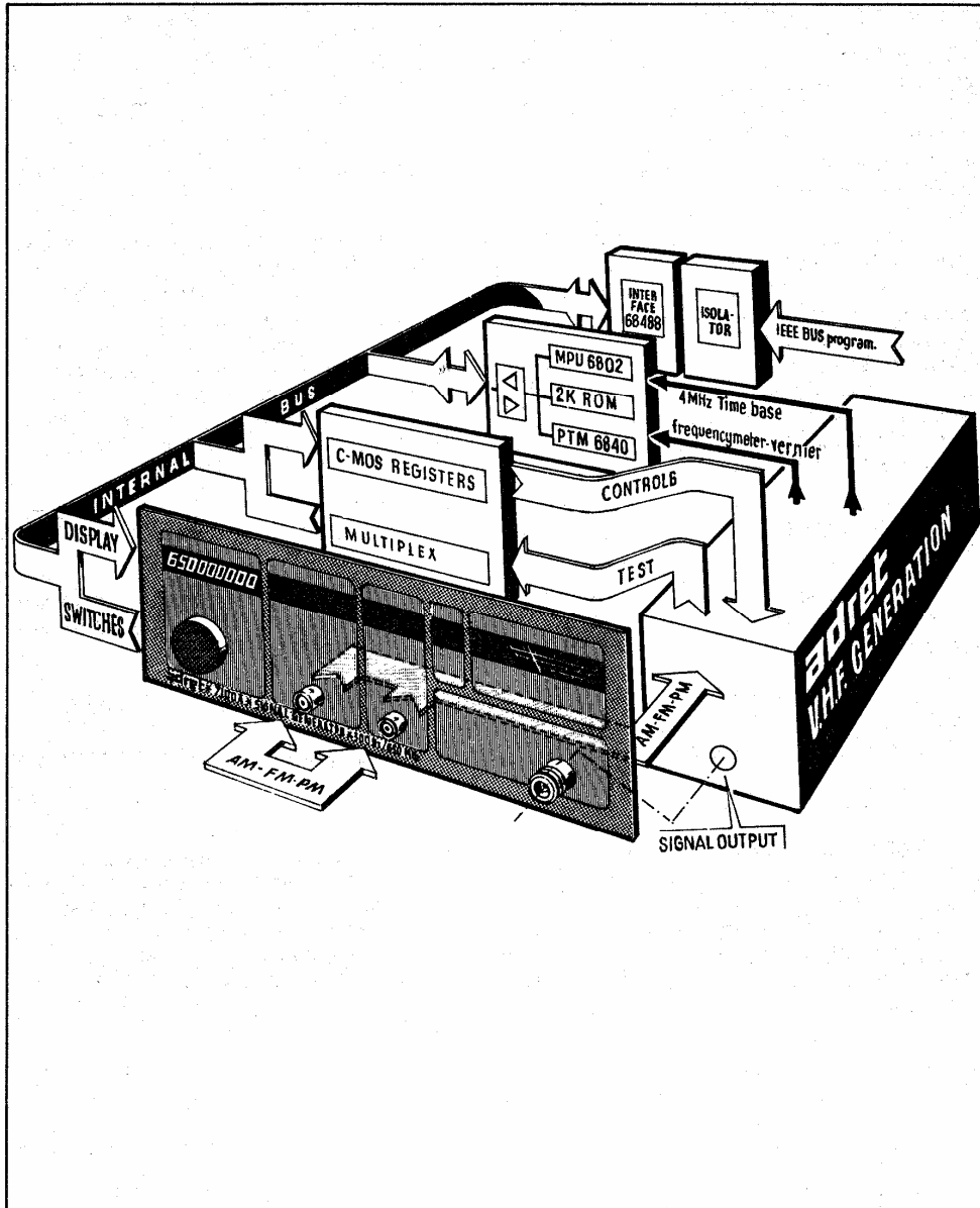
Figure 4-3 : GESTION PAR MICROPROCESSEUR
