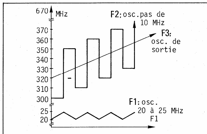
Figure 4-2 : PROGRESSION DES 3 OSCILLATEURS
