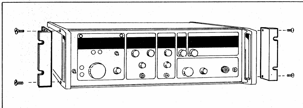
Figure 3-3 : MONTAGE DU 7100 EN RACK 19 POUCHES
