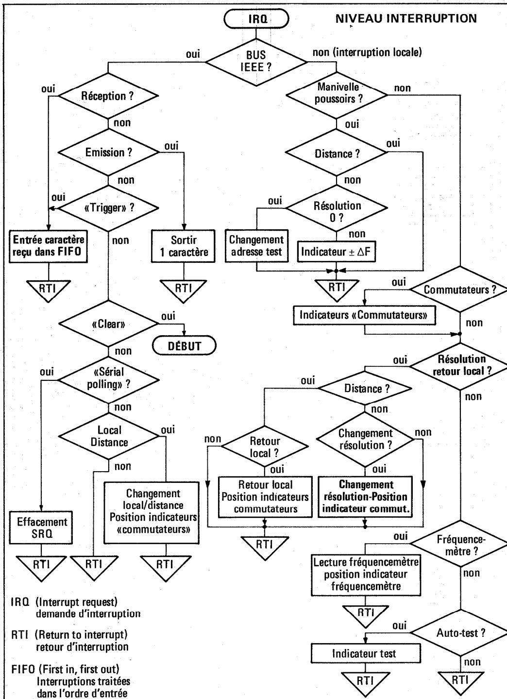
Figure 4-5 : ORDINOGRAMME DU MICROPROCESSEUR. NIVEAU INTERRUPTION
