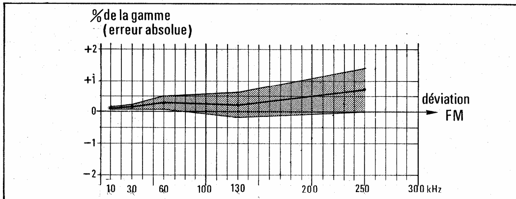
VALEURS MOYENNES ET ECARTS TYPE DE LA PRECISION DE LA DEVIATION FM Fréquence RF : 160 MHz ; Gamme de déviation : \pm 300 kHz ; Signal modulant de 400 Hz
