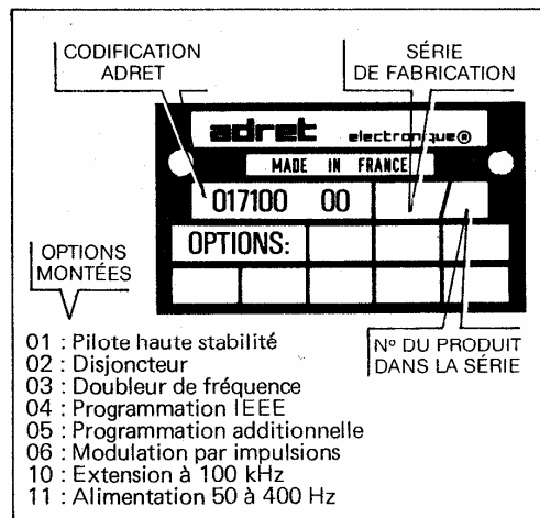
Figure 3-1 : CARACTERISATION DU GENERATEUR
