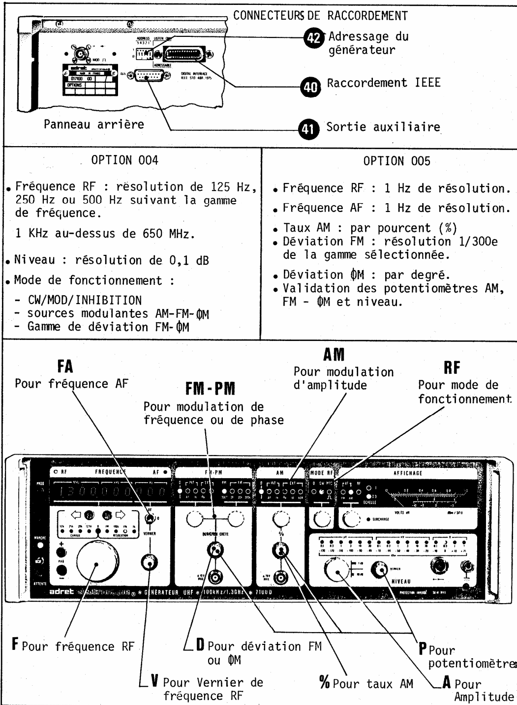
FIGURE 3 - 6 : DESCRIPTION DES OPTIONS DE PROGRAMMATION
