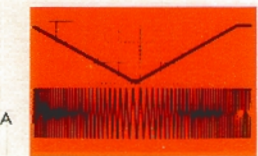
(A) Signal triangulaire et wobulation symétrique.
