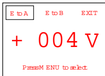
Abbildung 4 – Spannungsmeßanzeige
