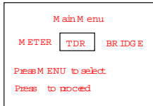
Afbeelding 3 - Hoofdmenu Display
