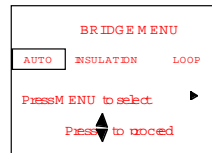
Abbildung 6 - Meßbrücken-Menü
