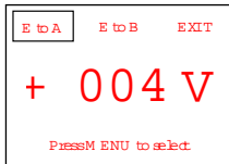
Afbeelding 4 – Voltmeter Display
