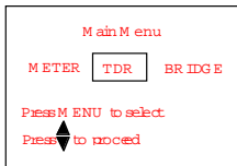
Abbildung 3 - Hauptmenüanzeige
