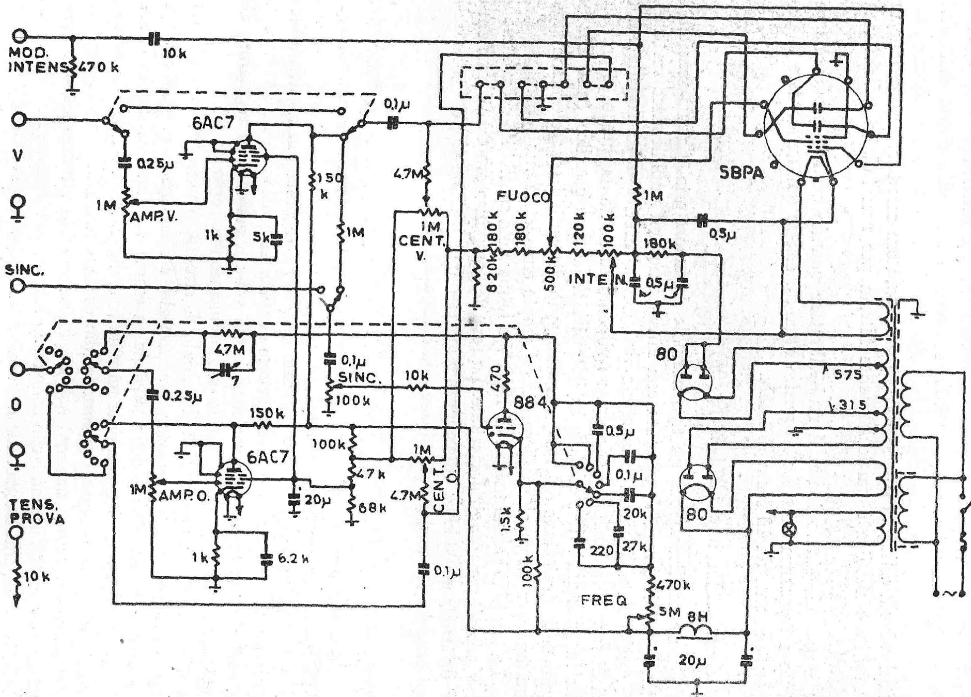
Fig. 96. - Oscilloscopio Du Mont 274-A.
