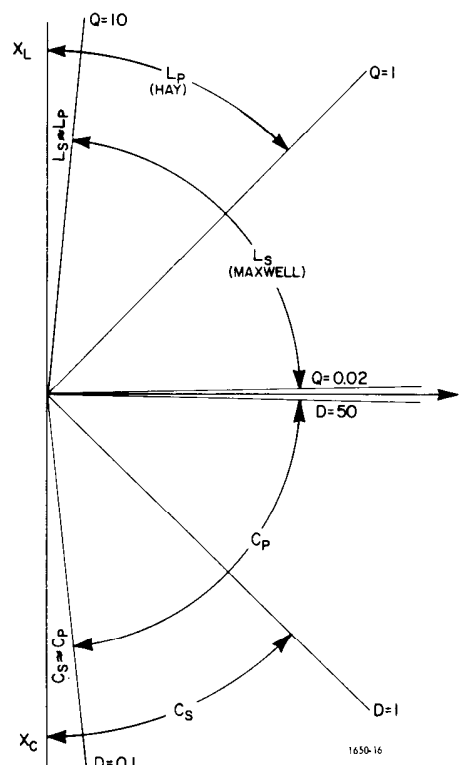
Figure 2-4. DQ coverage chart.
