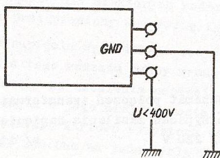
Rys. 5. Przyłożenie napięcia względem masy zasilacza.
