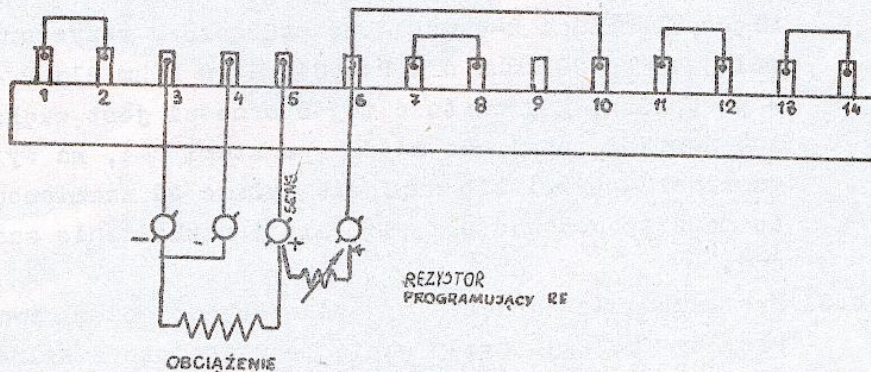
Rys. 11. Układ programowania prądu wyjściowego rezystorem zewnętrznym.
