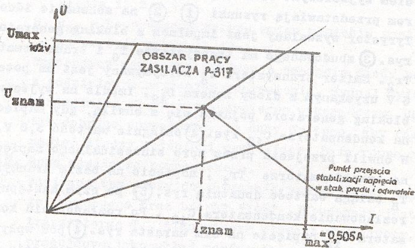
Rys. 1. Obszar pracy zasilacza P - 316, P - 317 / dla P - 316 U_{\text{maksymalne}} = 51 \text{ V} , I_{\text{maksymalne}} = 1 \text{ A} /
