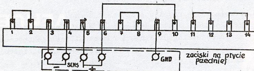
Rys. 7. Układ połączeń listwy na płycie tylnej przy samodzielnej pracy jednego zasilacza.
