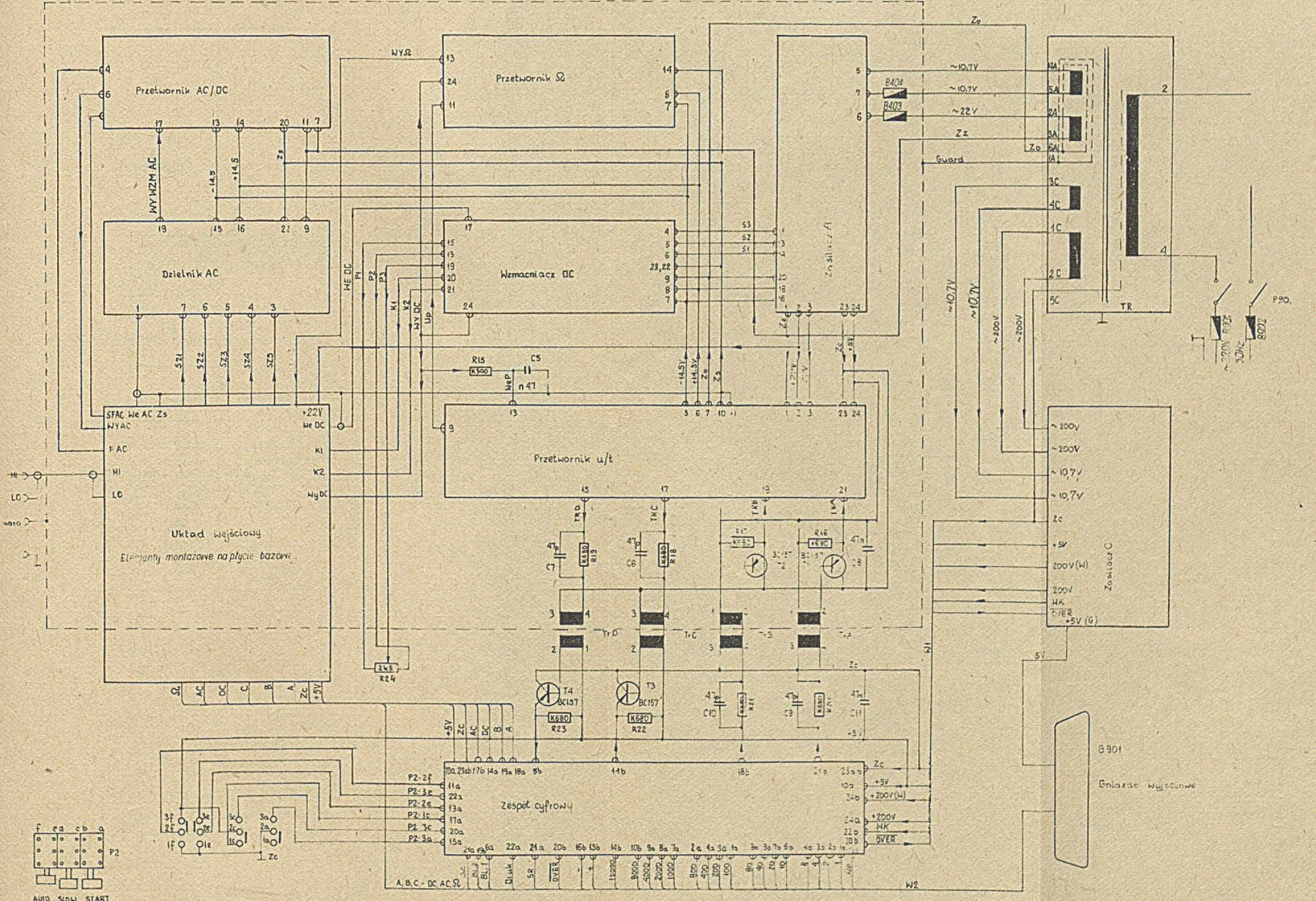
SCHEMAT OGÓLNY V543
