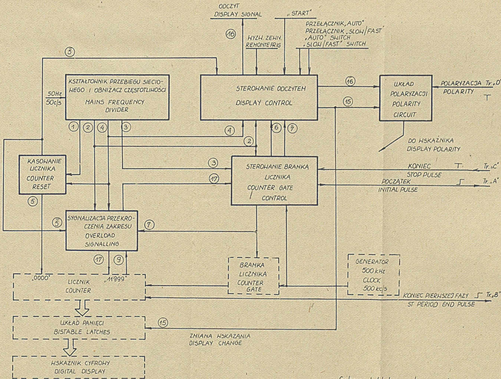
Schemat blokowy sterowania układu części cyfrowej
