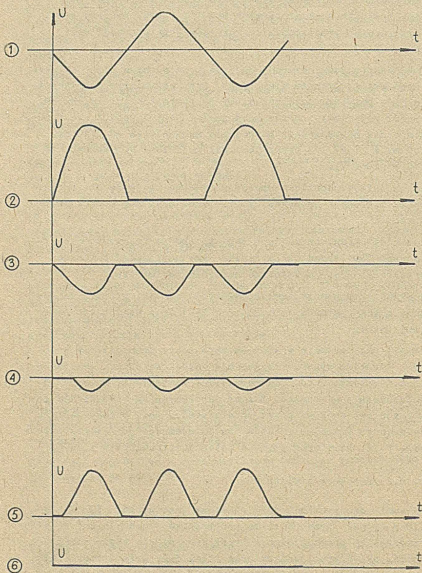
Przebiegi napięciowe w przetworniku AC/DC
