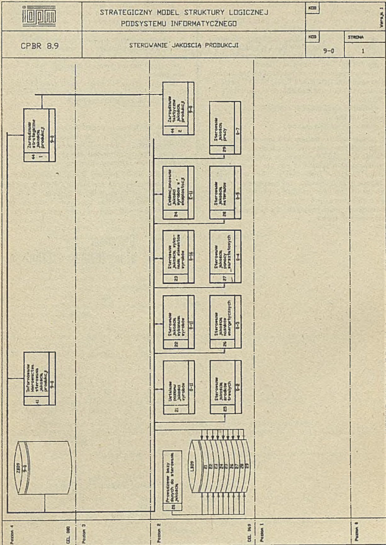
Rys. 22. Sterowanie jakością produkcji / cel 069/
