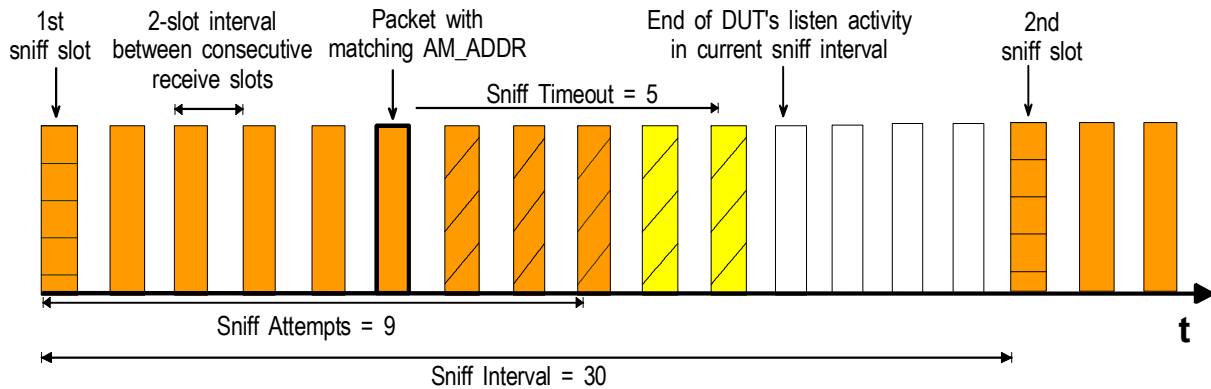
Fig. 4-96 Sniff mode parameters
