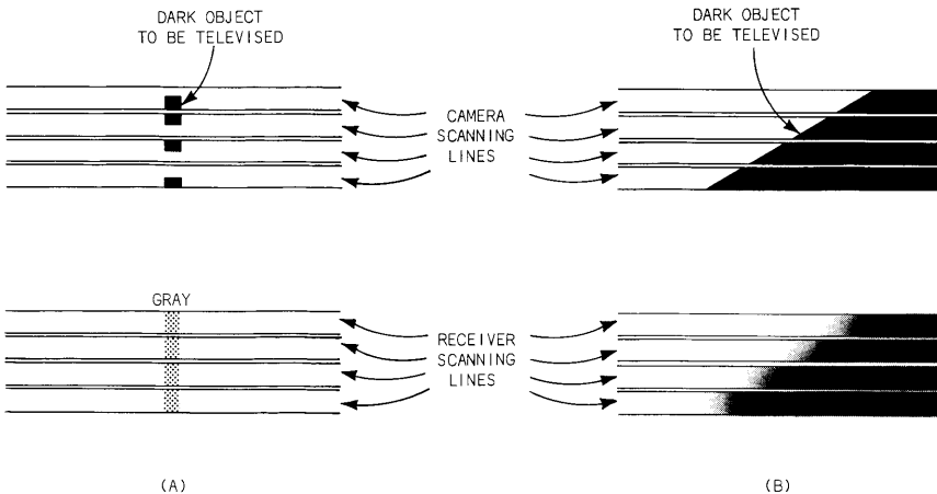
Fig. 9-9. Kell effect.
