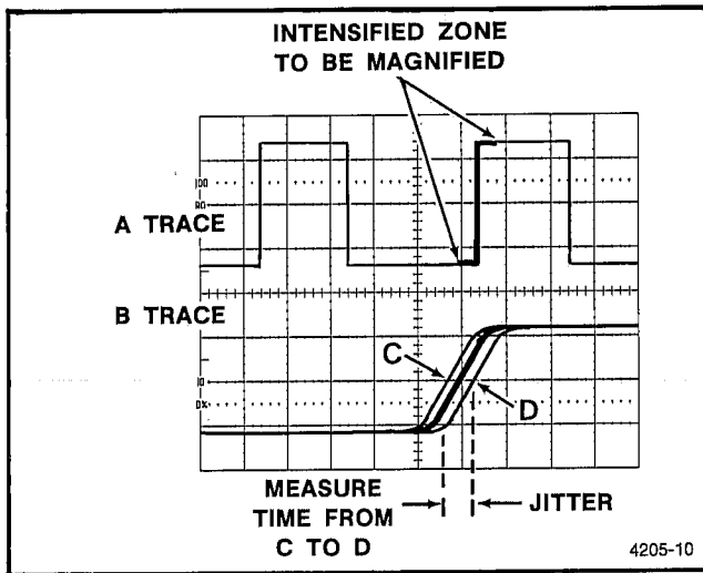
Fig. 4-6. Pulse jitter.
