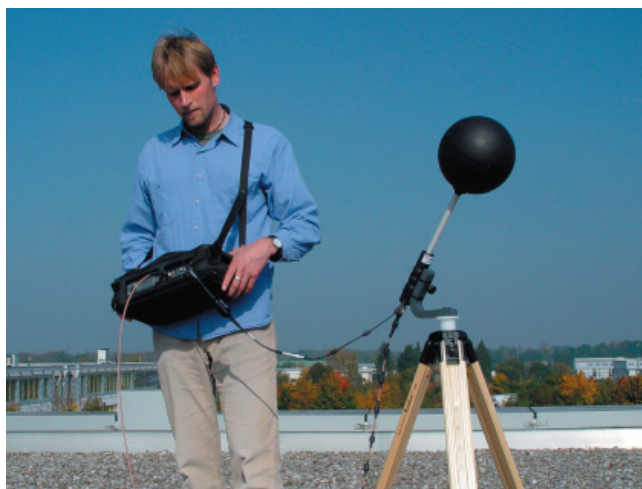
Messungen mit dem 9102 Handheld Spectrum Analyzer und der 9171 Isotropic Antenna
