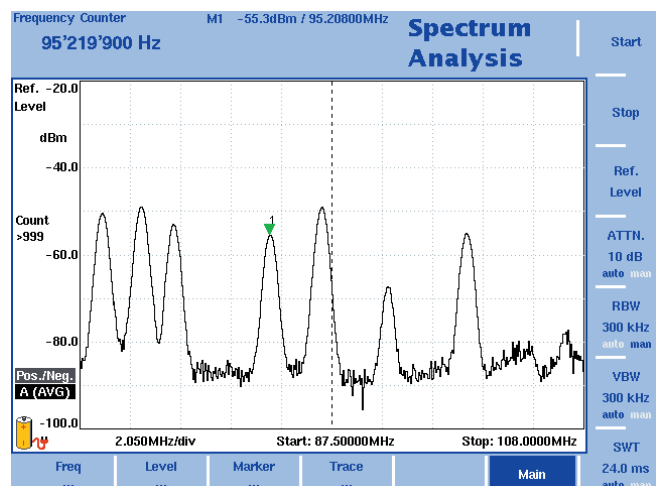
Exakte Frequenzkontrolle mit dem integrierten Frequenzzähler
