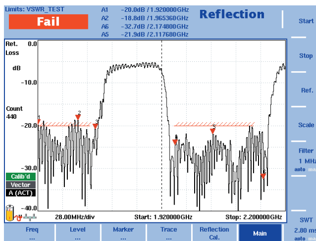
Prüfung von Antennensystemen auf einen Blick mit der Grenzwerttraster-Funktionalität. Der Fokus liegt auf der Rückflussdämpfung im Up- und Downlink.
