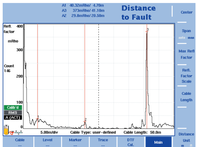
Präzise Ermittlung kleinster Kabelfehlstellen mit dem DTF-Modus im Feldeinsatz ...
