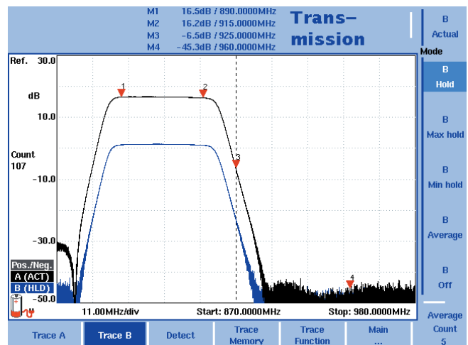
Messung der Verstärker-Kennlinie mit der Mitlaufgenerator-Option 9150
