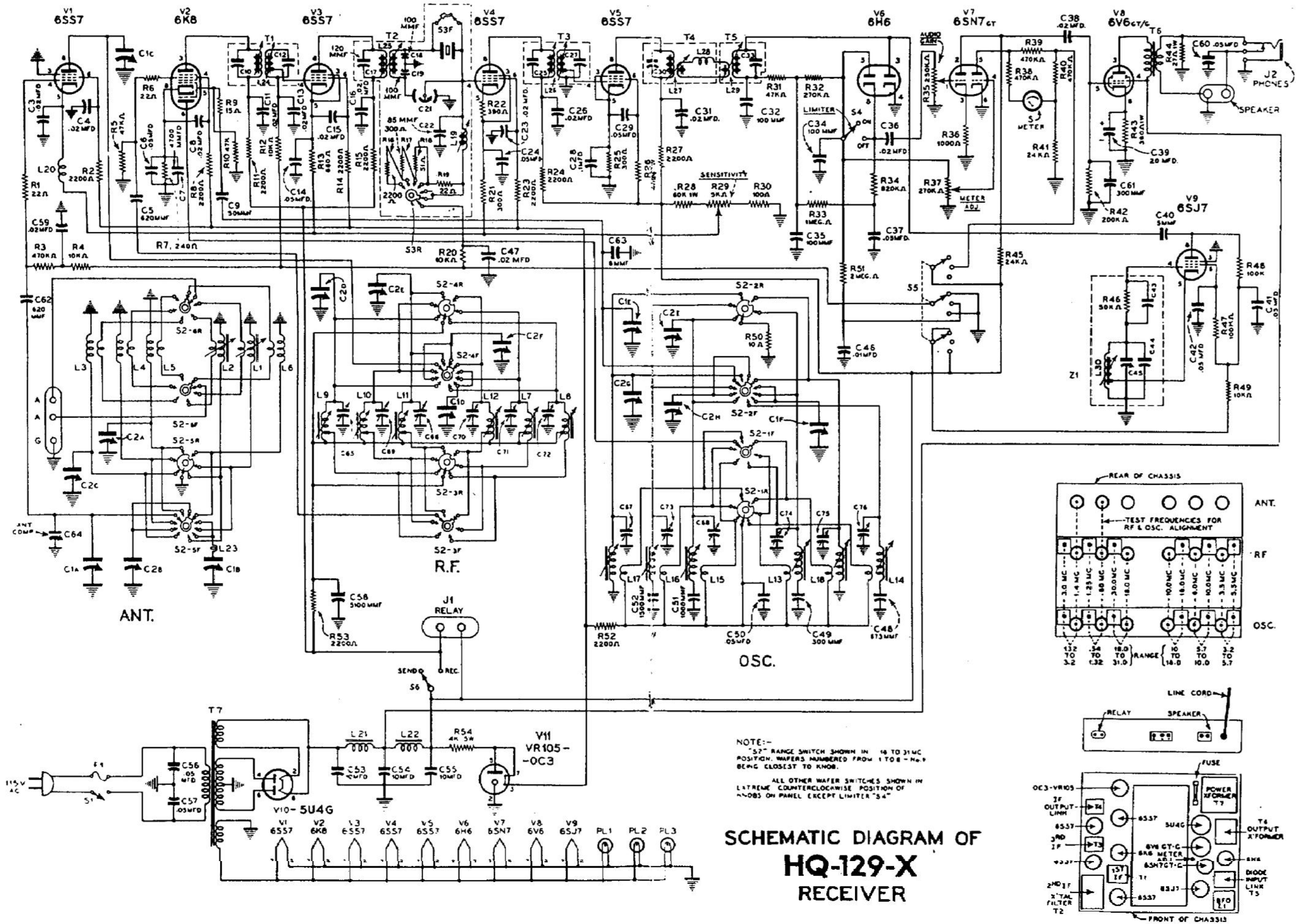
Fig. 8--Circuit diagram.
